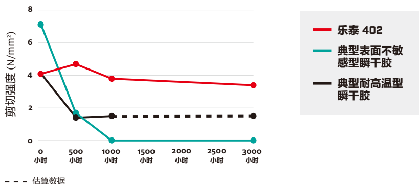
乐泰 402 VS. 其他典型瞬干胶： 在135°C下进行热老化后，测试135°C恒温条件下 胶粘剂在不锈钢基材上的剪切强度
