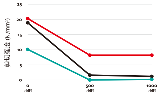
乐泰 402 VS. 其他典型瞬干胶： 在135°C下进行热老化后，测试恢复室温下 胶粘剂在不锈钢基材上的剪切强度
